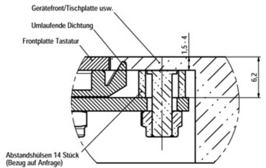
Einbauvorschlag Schnitt A-A (4 : 1)
