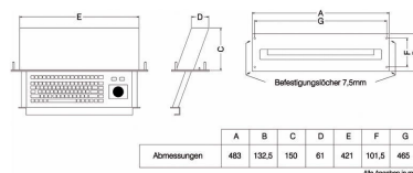
Geräteabmessungen:
