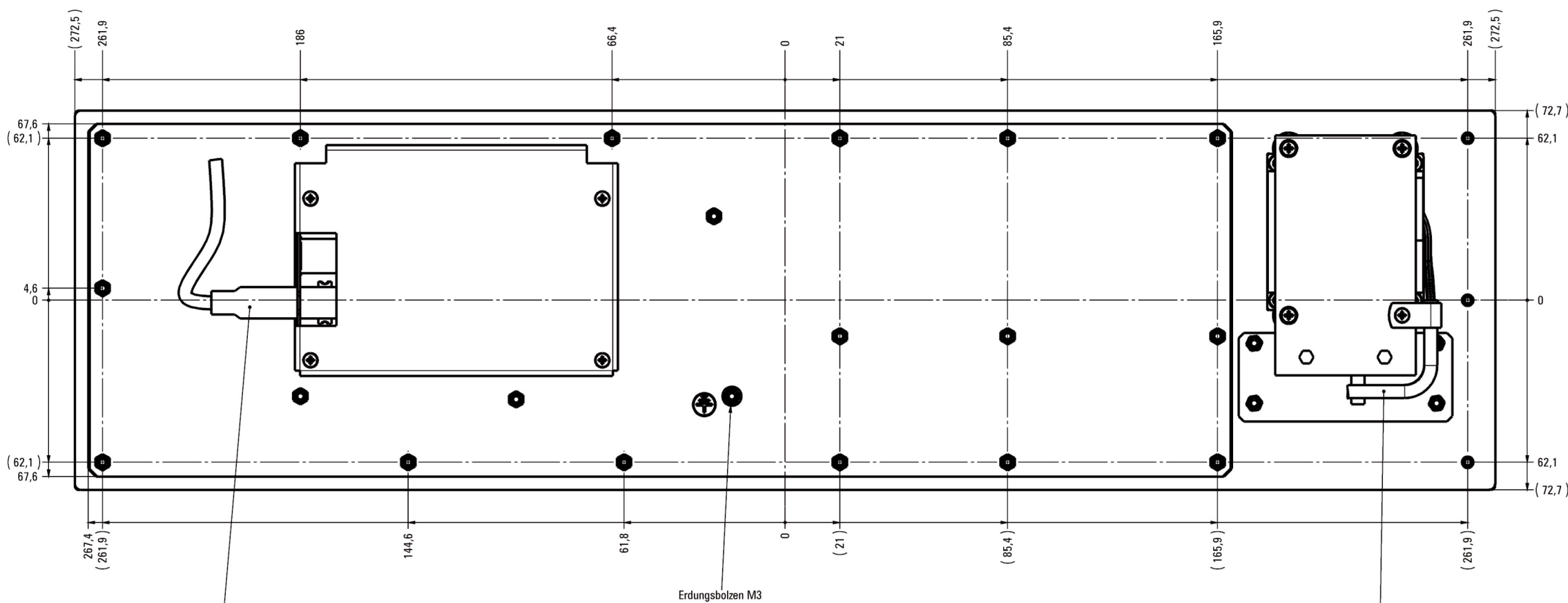
Erdungsbolzen M3
